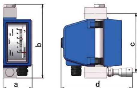
流向：侧进测出（带针阀）
