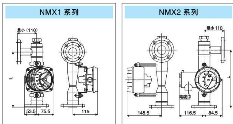
底侧(或底后侧)→顶侧(或顶后侧)外形图
